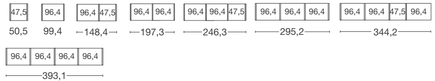
Drehtüreschrank Holztüren und Glas- oder Spiegeltüren mit Querriegel
