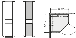
Ausgebauter Eckschrank, wahlweise mit Holz-, Spiegel- oder Glastür, mit Querriegel, inkl. Kranzleiste
